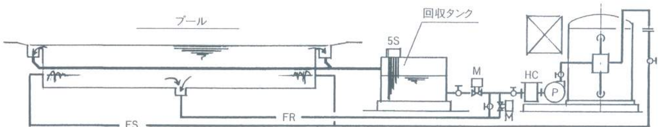
プール用オーバーフロー回収濾過設備フローシート
